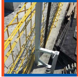
Kiriş Sıkıştırırmalı Dikme Beam Compressible Post Poste à Poutre Compressible
